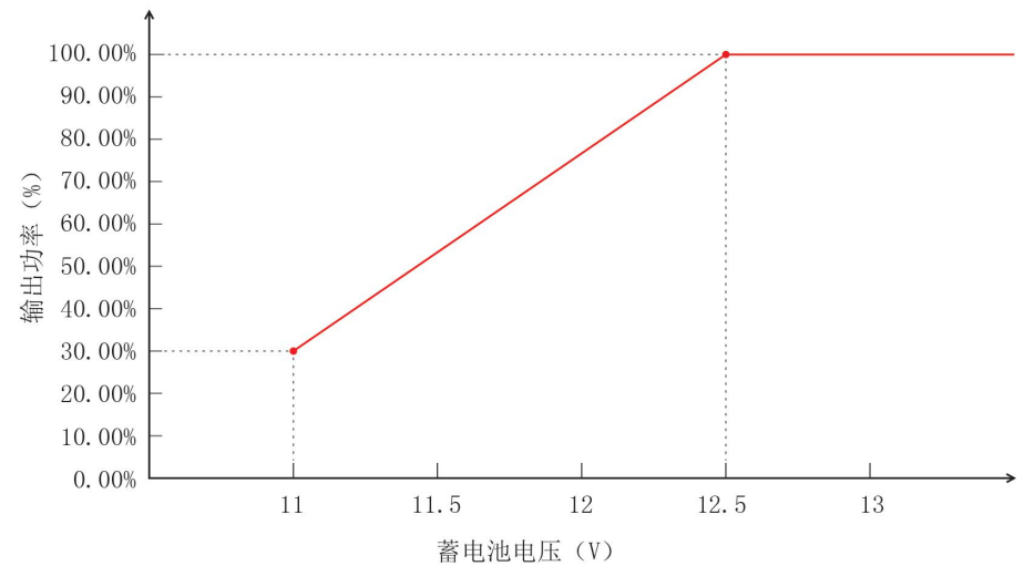
蓄电池电压VS输出功率
